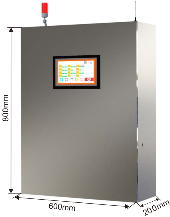
图 1 产品外观图
